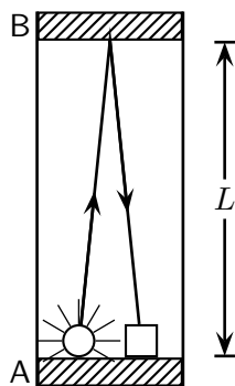
Figur 3.3: Feynman-uret.
